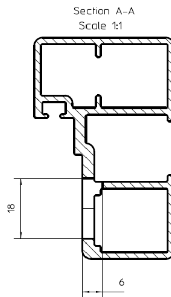
HK3101: Doorframe
